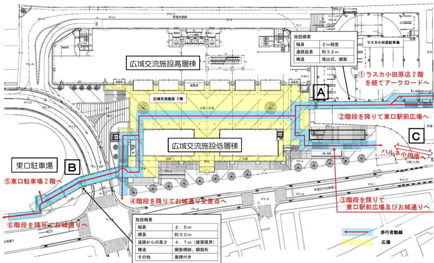
図1 広域交流施設と小田原駅周辺施設の接続(案)
