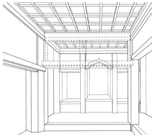
図1 摩利支天を祀る空間の復元パース
