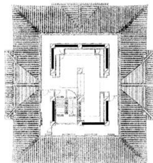
3階平面図
