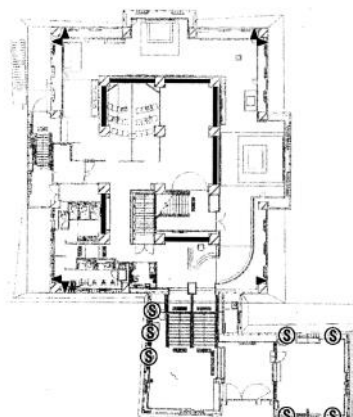
1階平面図
