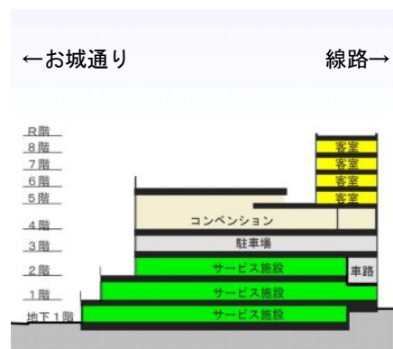
図2 施設棟断面図
