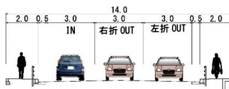
横断図 2 (市道 4 6 4 3)
