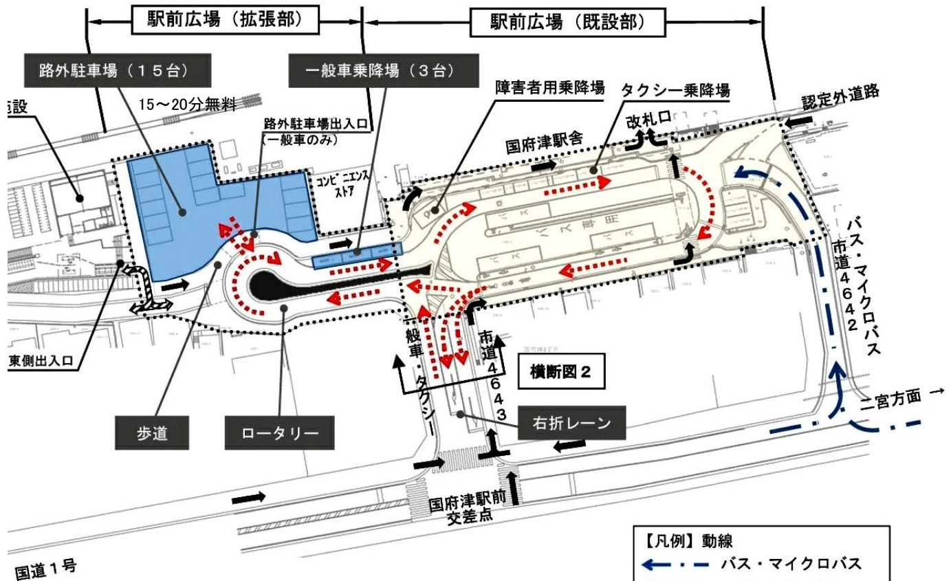
横断図 2 (市道 4 6 4 3)
