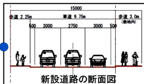
新設道路の断面図
