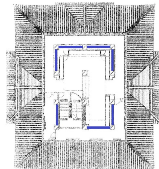
3階平面図
