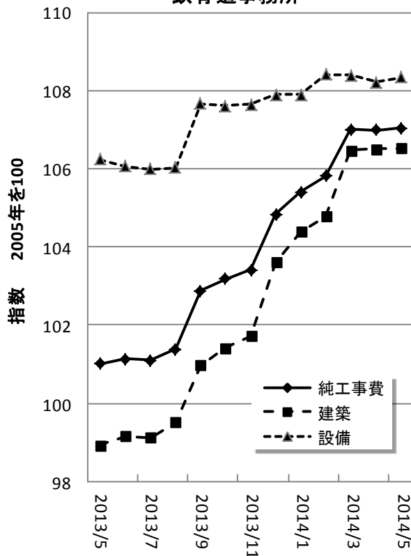
図1 2005年を100とした建設指数の推移 鉄骨造事務所
