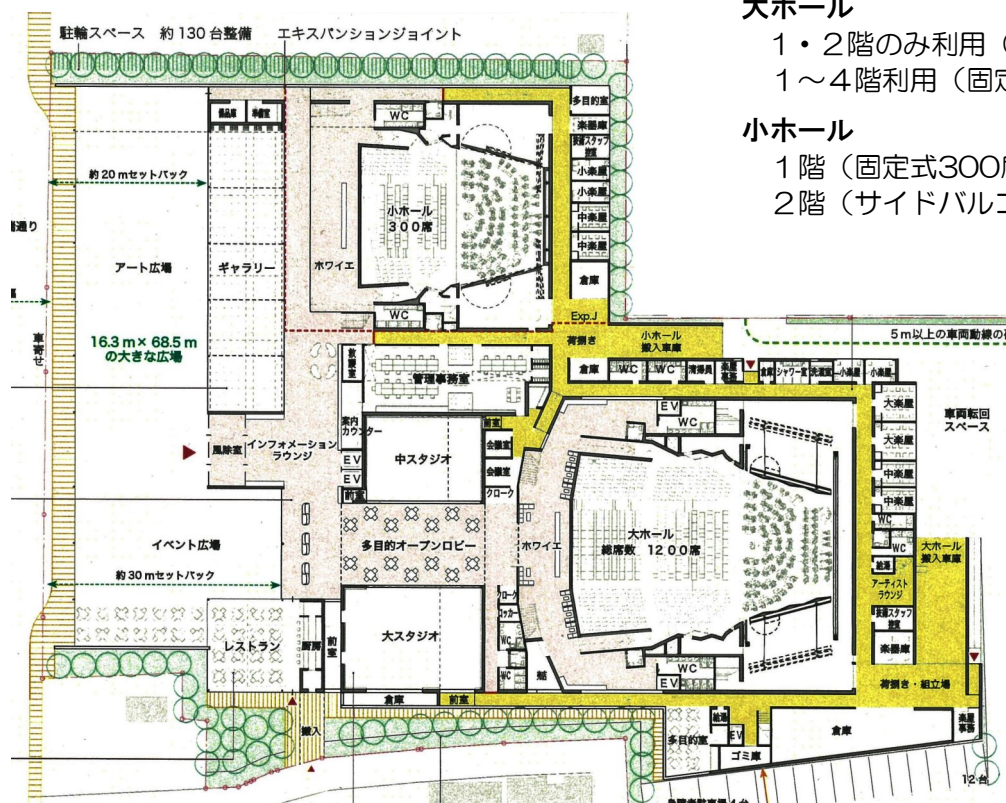
▲図4 芸術文化創造センター1階 設計提案図
