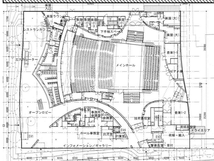
▲図3 城下町ホール1階設計図
