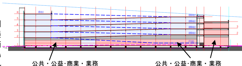
図2 駐車場施設断面図イメージプラン
